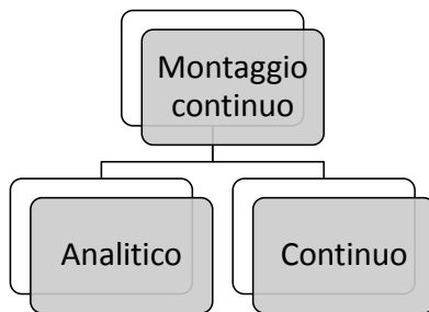
Continuità spazio-tempo
