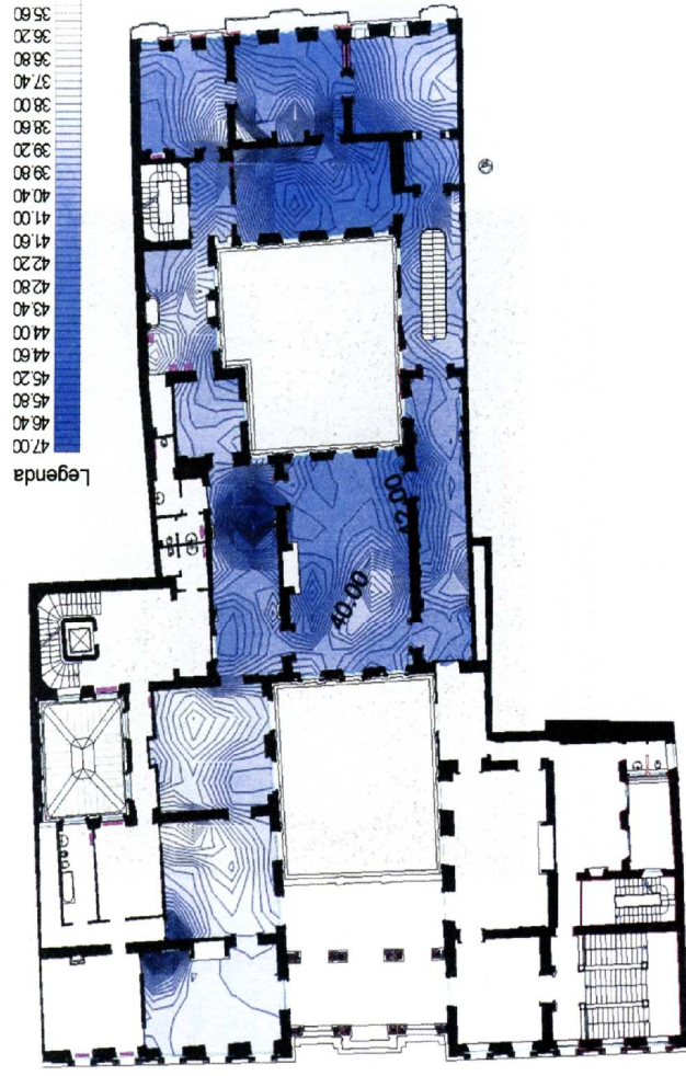
Immagine 14 – Palazzo Bagatti Valsecchi, Milano. Mappatura dell'umidità relativa all'interno del primo piano rilevata alle ore 15, mediante l'utilizzo di psierometro digitale.
