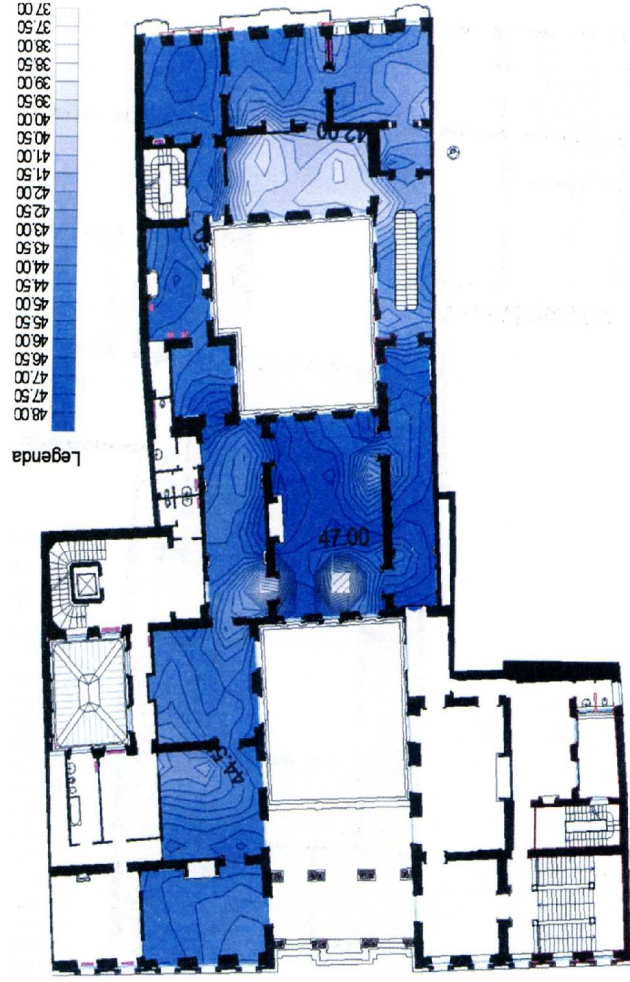
Immagine 13 – Palazzo Bagatti Valsecchi, Milano. Mappatura dell'umidità relativa all'interno del primo piano rilevata alle ore 9,45, poco dopo l'accensione dell'impianto di riscaldamento, mediante l'utilizzo di psicrometro digitale.
