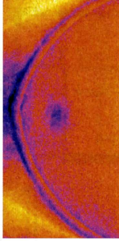
Immagine 10 – Abbazia di Viboldone, San Giuliano Milanese (MI). Interno della chiesa. La ripresa termografica della parete (range 15,5-17,8 °C) con l'affresco della Madonna in trono evidenzia un "ponte termico", dovuto al tamponamento di un'apertura posta al centro della parete, in corrispondenza della quale possono verificarsi fenomeni di degrado causati dalla differente inerzia termica dei materiali che costituiscono il tamponamento stesso. Termografia eseguita dal laboratorio del Dipartimento di Conservazione e Storia dell' Architettura del Politecnico di Milano.
