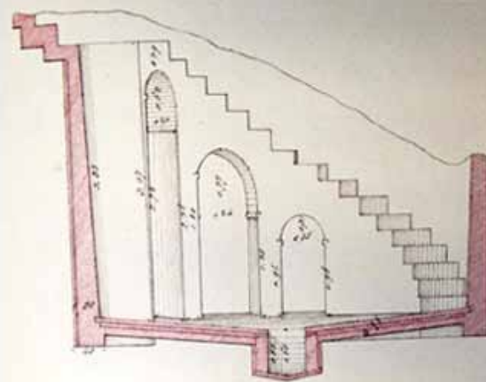
Prospetto della scala
