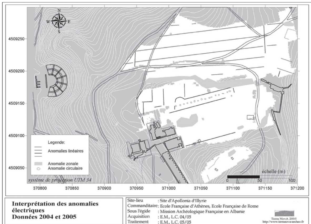
Fig. 4 - Interprétation des anomalies électriques (M. Dabas).
